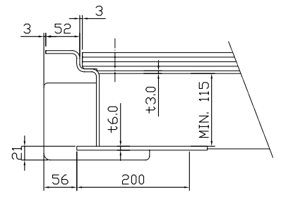
SECTION D-D 1:10
